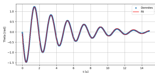
Figure 14: Mesure de l'angle \theta à 0.5A
