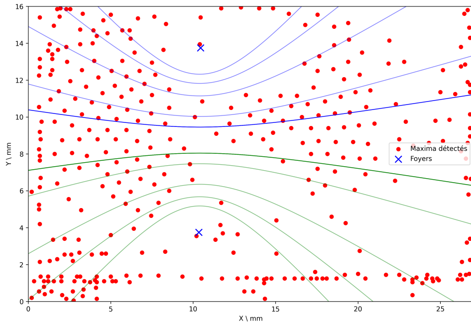
FIGURE 13 – image post-traitement sans superposition a l'échelle
