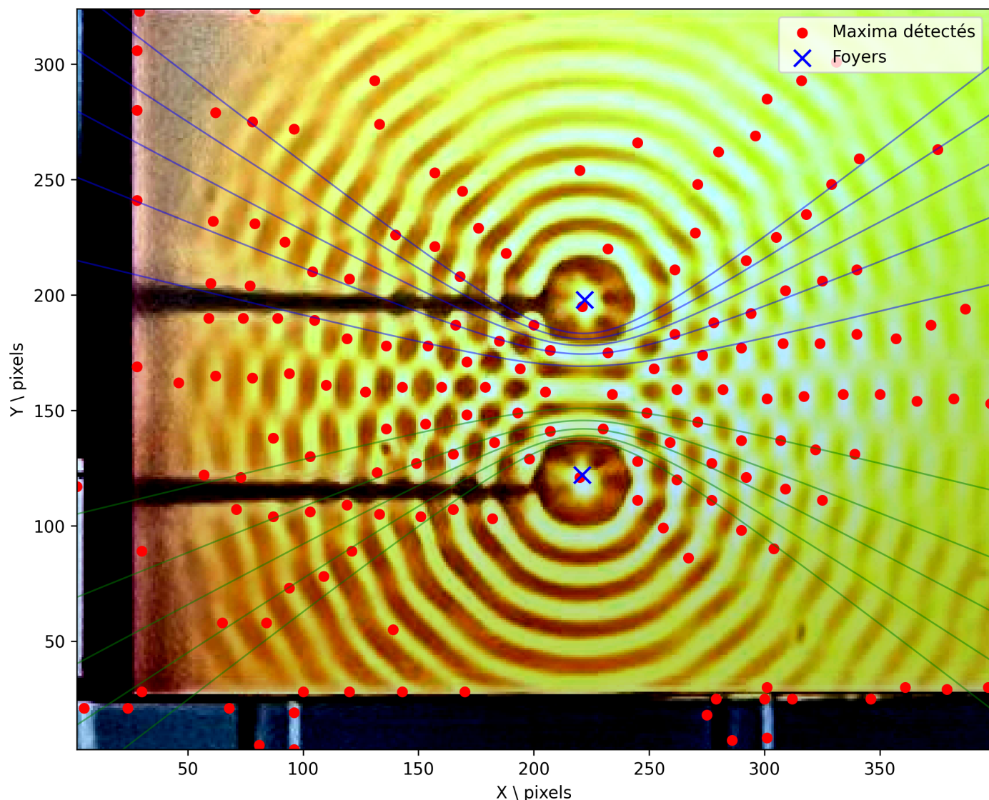
FIGURE 7 – Excitation à 25.2 \pm 0.5 Hz avec D = 41 \pm 1 mm entre excitateurs
