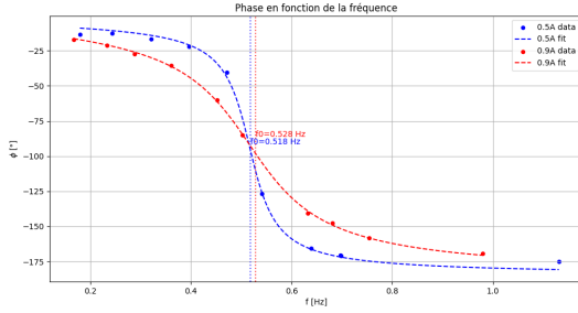
Figure 6: Phase en fonction de la fréquence
