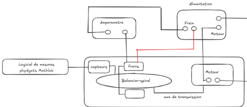
Figure 2: Schema electrique pour la prise de mesure en regime d'oscillations libres
