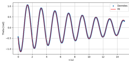
Figure 13: Mesure de l'angle \theta à 0.3A
