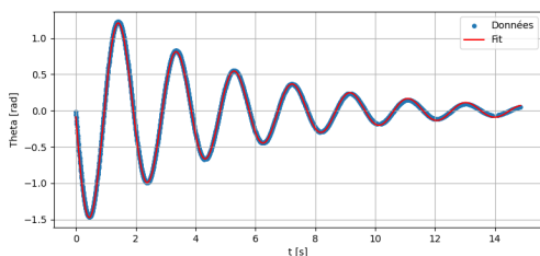
Figure 15: Mesure de l'angle \theta à 0.5A
