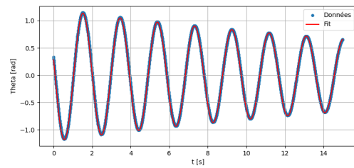
Figure 10: Mesure de l'angle theta a 0.2A
