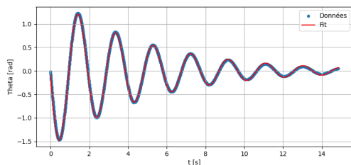
Figure 13: Mesure de l'angle theta a 0.5A
