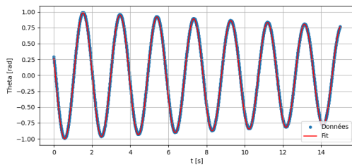
Figure 9: Mesure de l'angle theta a 0.1A
