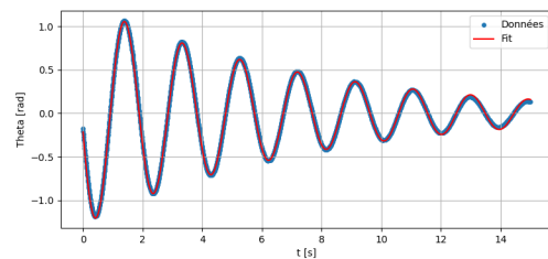
Figure 12: Mesure de l'angle theta a 0.4A
