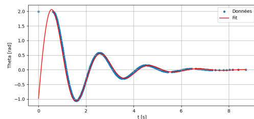
Figure 14: Mesure de l'angle theta a 0.9A
