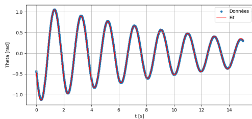
Figure 11: Mesure de l'angle theta a 0.3A
