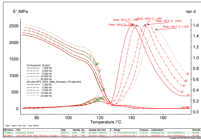
Figure 5: Analyse du pic de \tan \delta permettant l'extraction de T_g(f)
