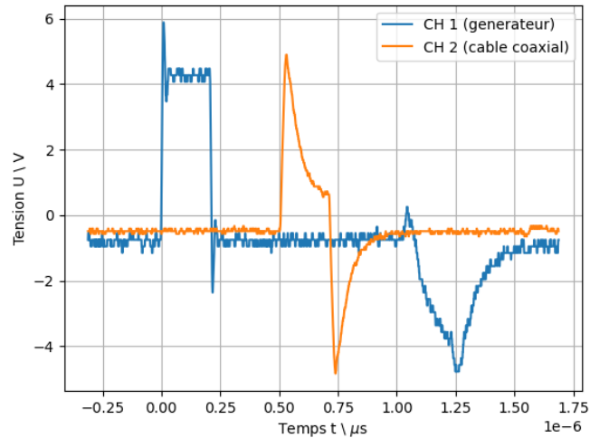
Figure 8: Mesure des impulsions de largeur (width) w = 210 \text{ ns}
