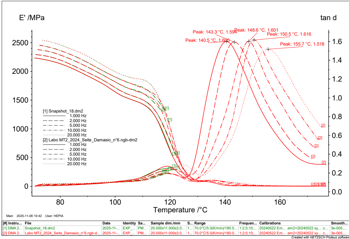
Figure 3: Analyse du pic de \tan \delta permettant l'extraction de T_g(f)
