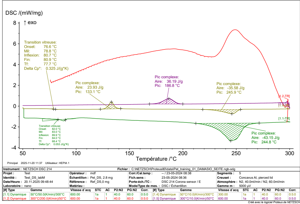
Figure 11: Vue d'ensemble des mesures DSC
