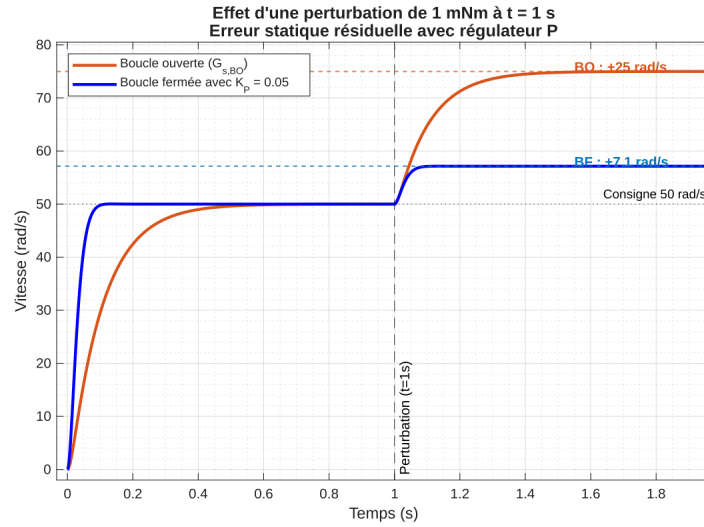
FIGURE 9 – Effet de la perturbation de 1 mNm à t = 1 s en BO et BF. BF : déviation \approx +7,1 rad/s. BO : déviation \approx +25 rad/s.
