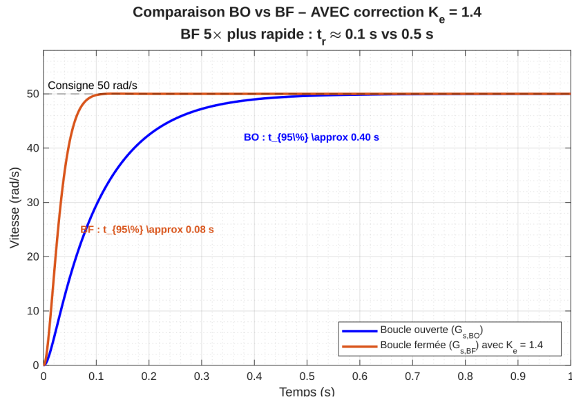
FIGURE 7 – Comparaison BO (bleu) vs BF (orange) avec correction K_e = 1.4 . Les deux atteignent 50 rad/s, mais la BF est 5× plus rapide ( t_r \approx 0.1 s vs 0.5 s).
