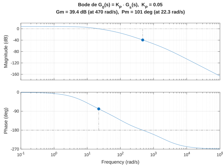
FIGURE 10 – Diagramme de Bode de G_0(s) = K_P \cdot G_s(s) avec K_P = 0,05 . PM = 101° à \omega_c = 22,3 rad/s, GM = 39,4 dB à 470 rad/s.
