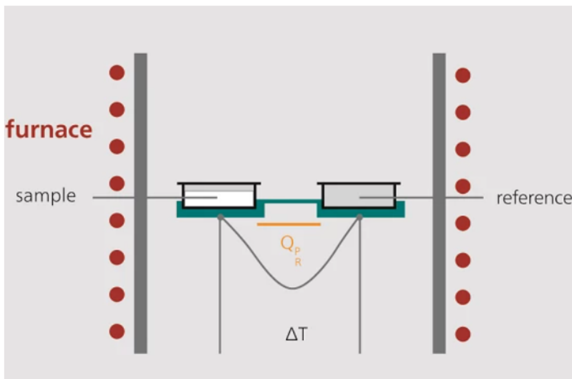
Figure 6: Schéma de principe de la mesure DSC, Ref. [3]
