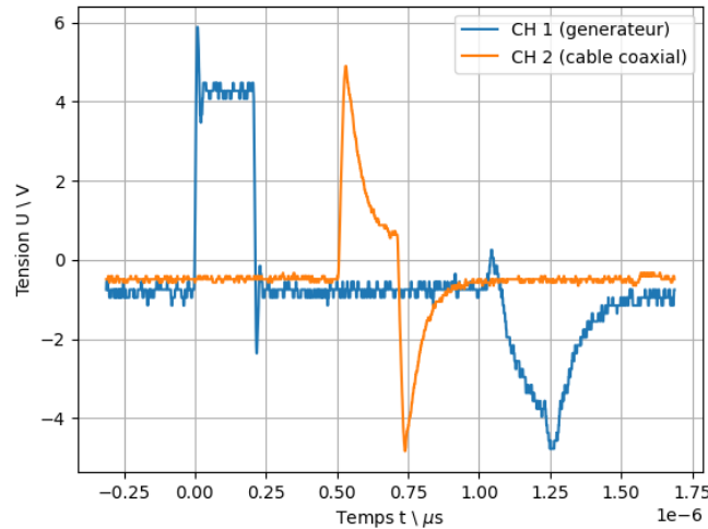
Figure 9: Mesure des impulsions de largeur (width) w = 210 \text{ ns}
