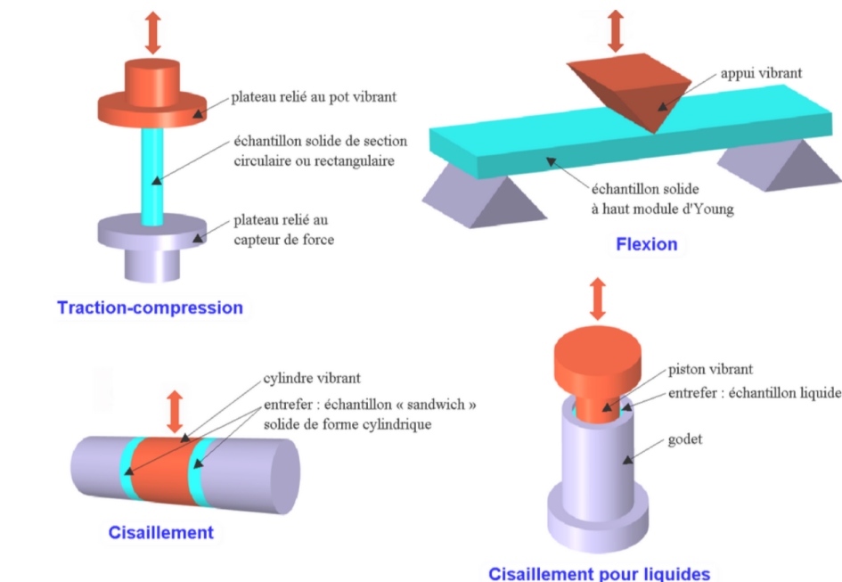
Figure 1: Techniques d'analyses des proprietes mecaniques d'un solide, ref : [1]
