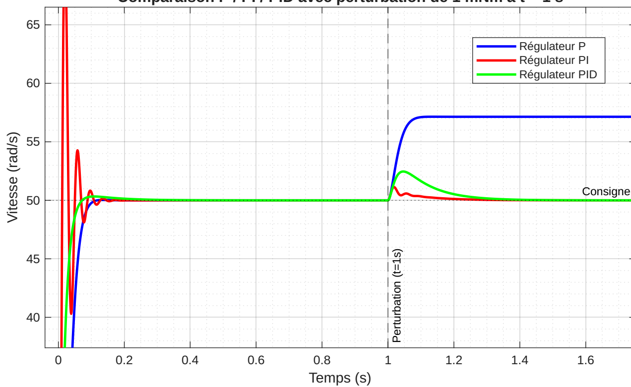
Comparaison P / PI / PID avec perturbation de 1 mNm à t = 1 s
