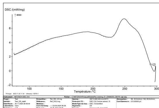
Figure 7: \delta H(T[^\circ\text{C}]) refroidissement rapide
