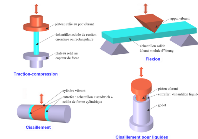
Figure 1: Techniques d'analyse des propriétés mécaniques d'un solide, réf. : [1]
