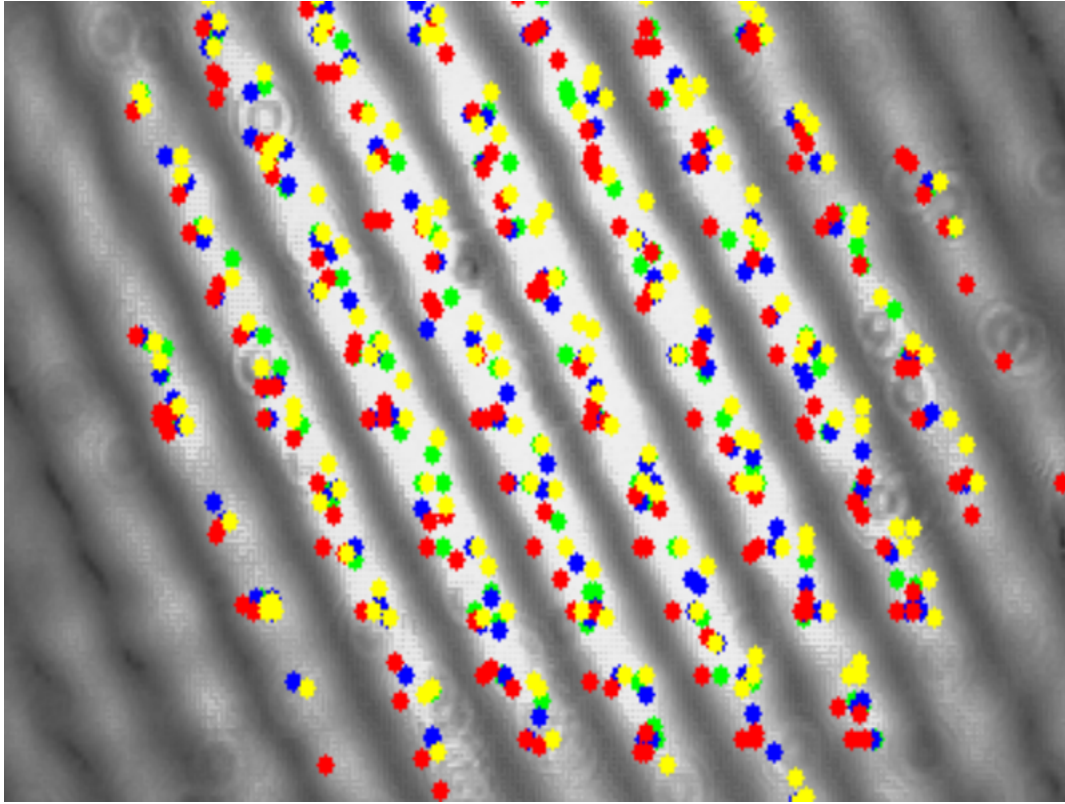
Figure 10: Superposition des figures d'interferometries pour 5V (vert), 10V (bleu), 15V (rouge) et 20V (jaune)
