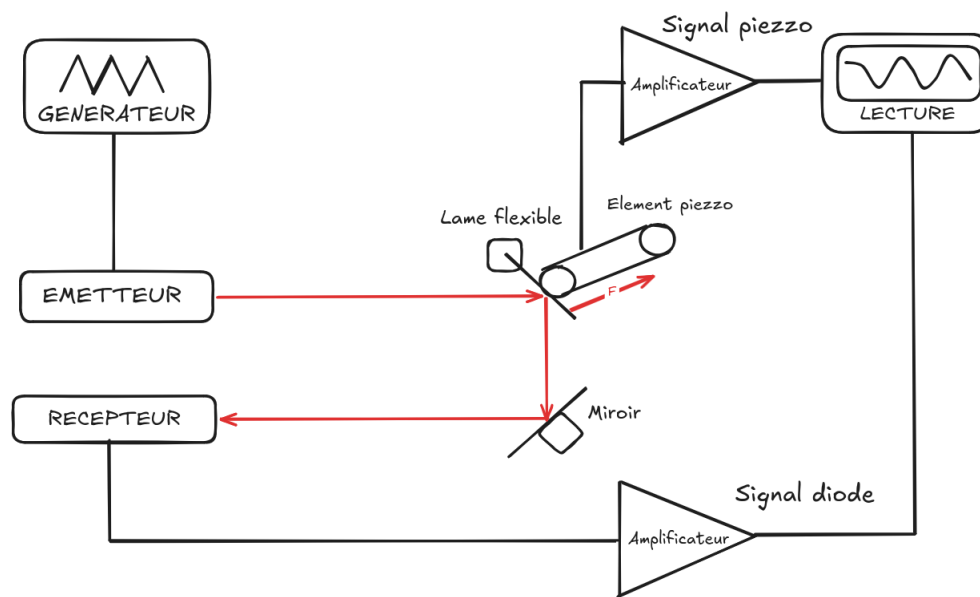
Figure 1: Schéma du dispositif de mesure de l'hysteresis
