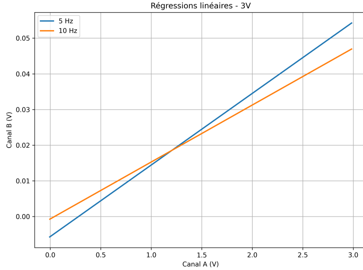
Figure 6: d(V) pour 3V
