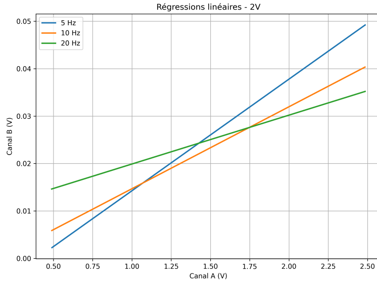
Figure 5: d(V) pour 2V
