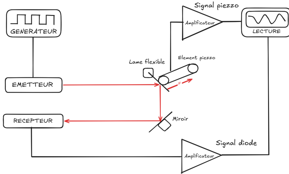
Figure 2: Schema du dispositif de mesure du fluage
