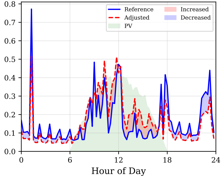
Prosumer B (Medium PV)
