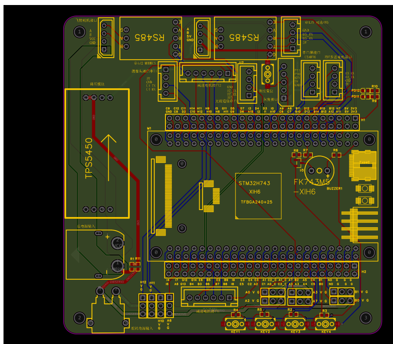
图 3.8 自动循迹底盘电路 PCB 布局
