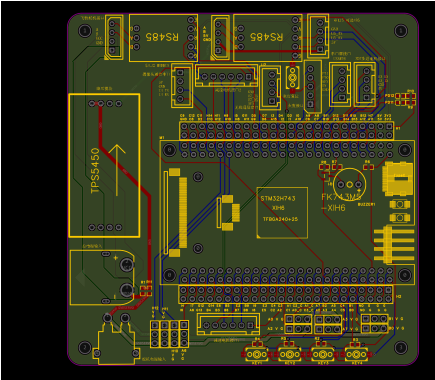
(b) 瞄准模块电路 PCB 布局
