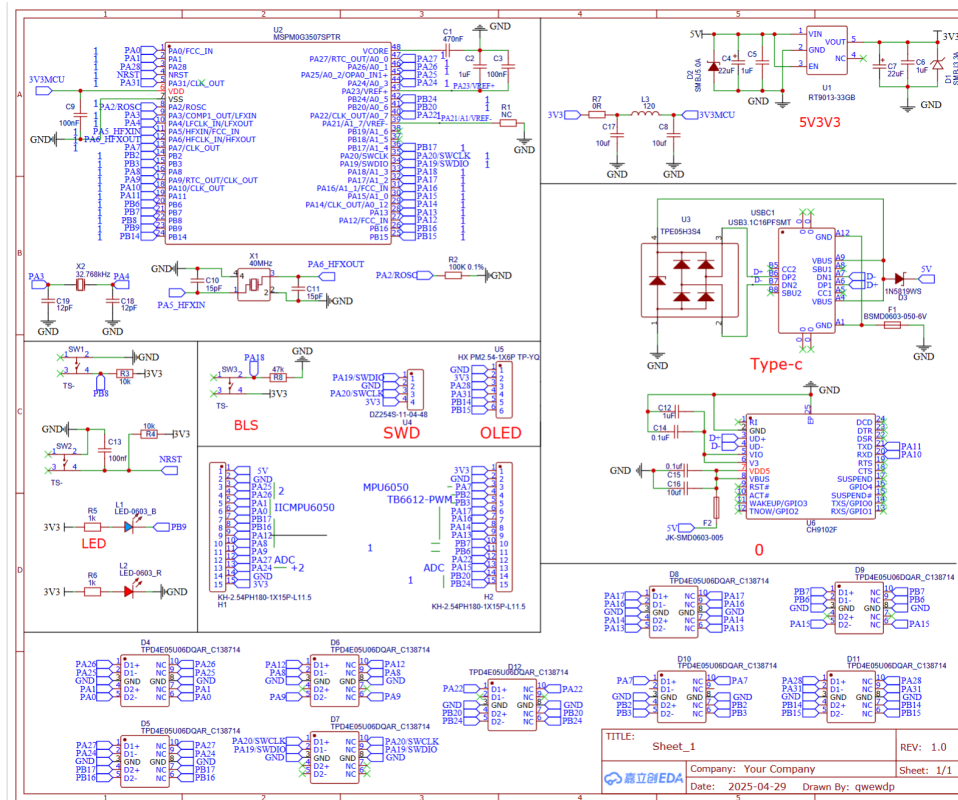
(a) 自动循迹底盘电路原理图
