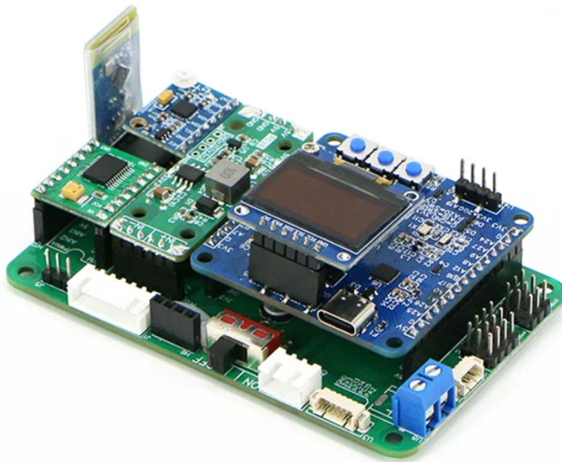
(b) 自动循迹底盘电路 PCB 实物图
