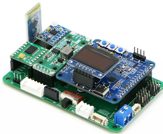
图 3.8 自动循迹底盘电路 PCB 实物图
