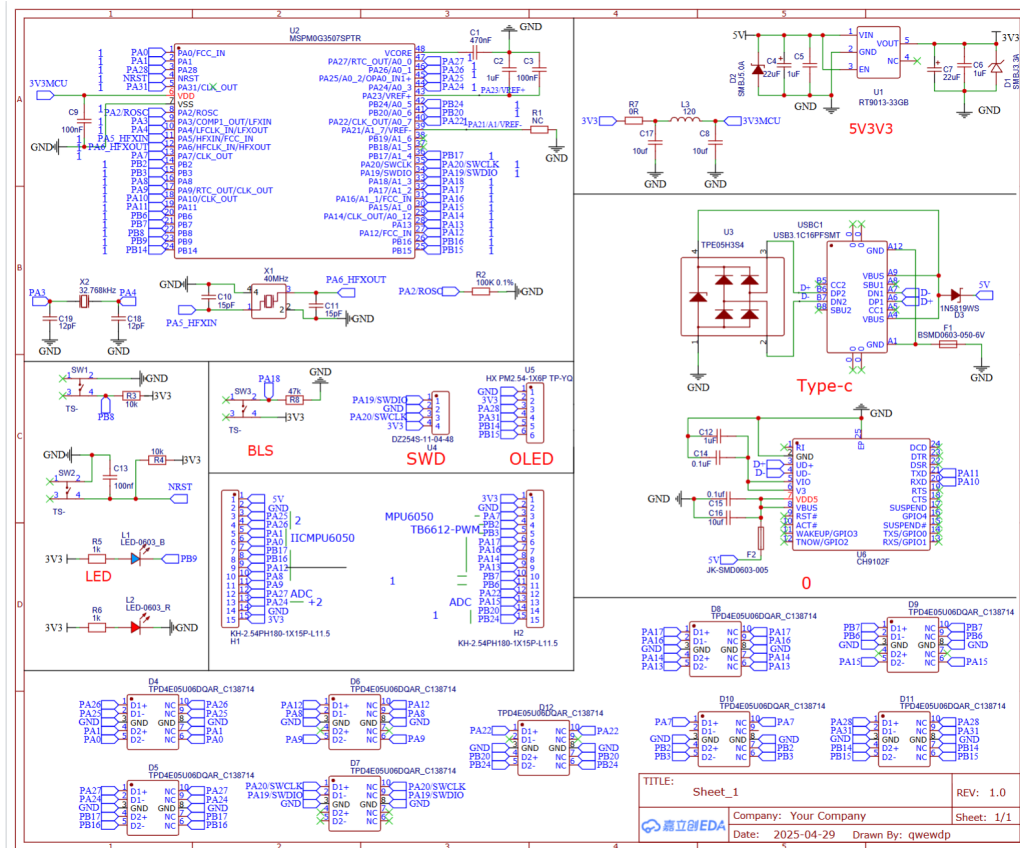
图 3.7 自动循迹底盘电路原理图
