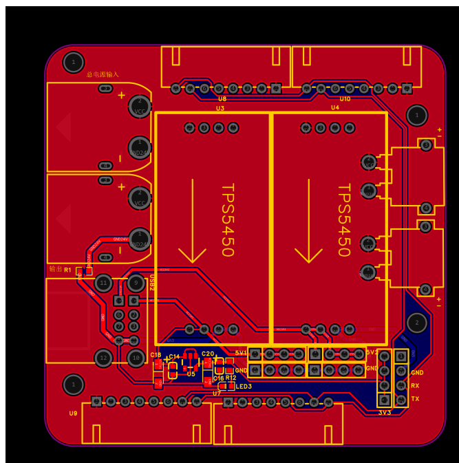
图 3.6 电源电路 PCB 布局
