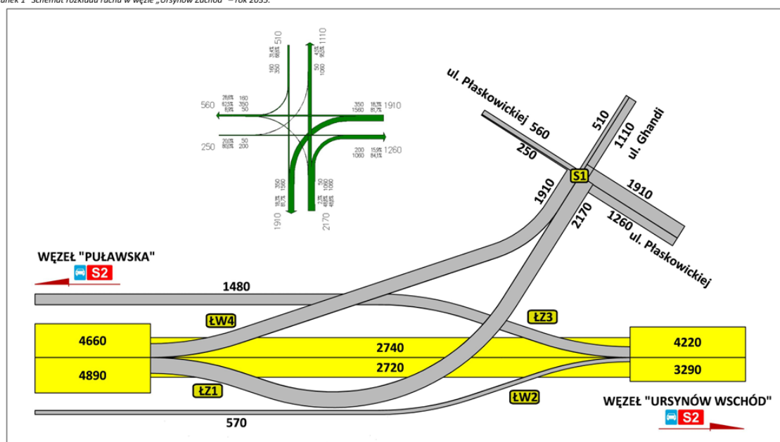
Analiza przepustowości odcinków międzywęzłowych, obszarów wyłączania i włączania na łącznicę/z łącznic oraz łącznic i skrzyżowań dla Południowej Obwodnicy Warszawy od węzła „Puławska” do węzła „Lubelska” Rysunek 1 Schemat rozkładu ruchu w węźle „Ursynów Zachód” – rok 2035.
