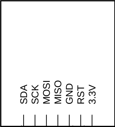
RFID RC522 Module
