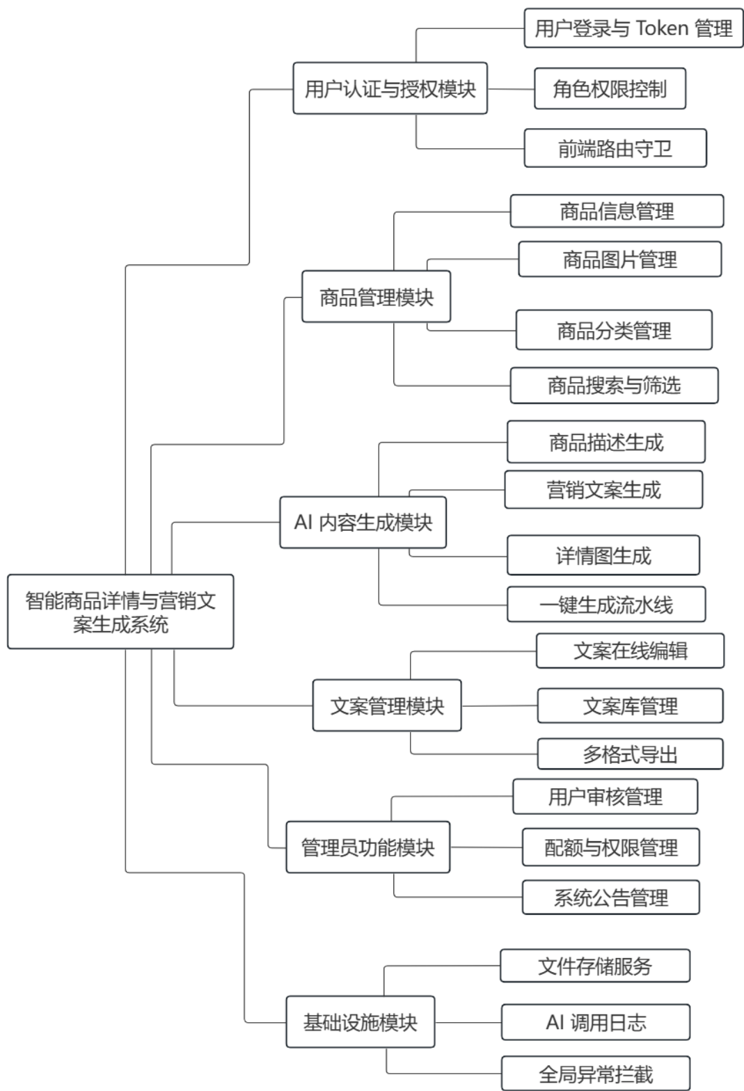
图 2 系统功能模块结构图
