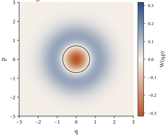
25. Wigner function
