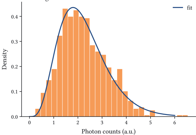
26. Histogram
