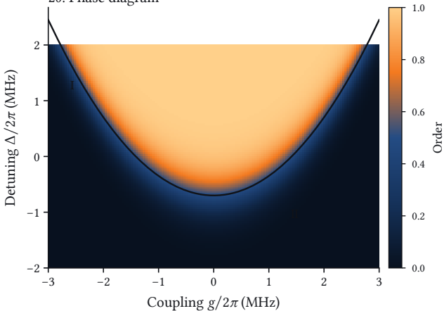
20. Phase diagram
