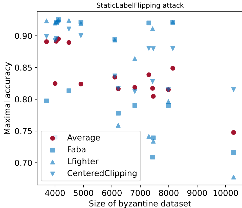
dirichlet_niid_modified, 0.05
