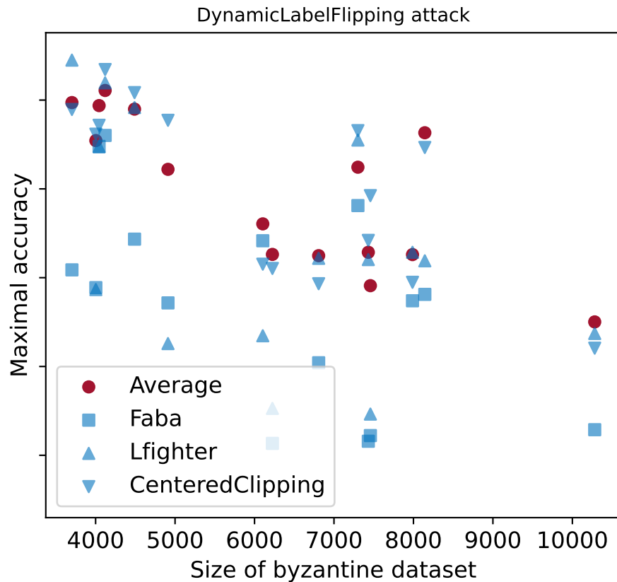
dirichlet_niid_modified, 0.05
