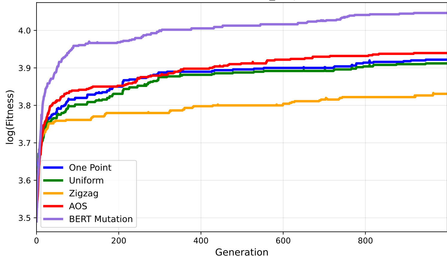
Artificial Ant (aux_map2)
