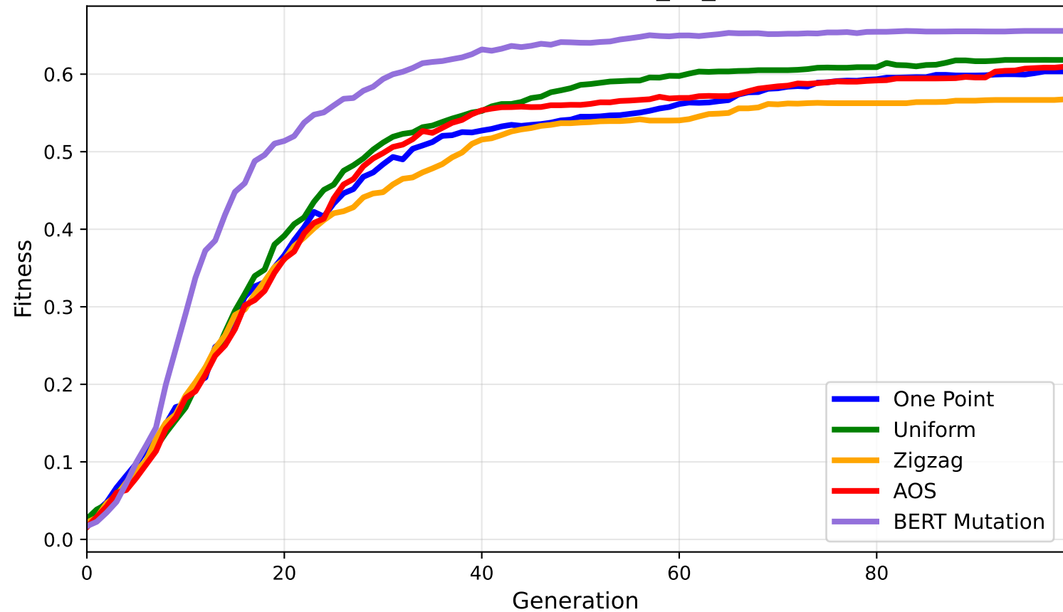
Frozen Lake (rand8x8_2k_eval)
