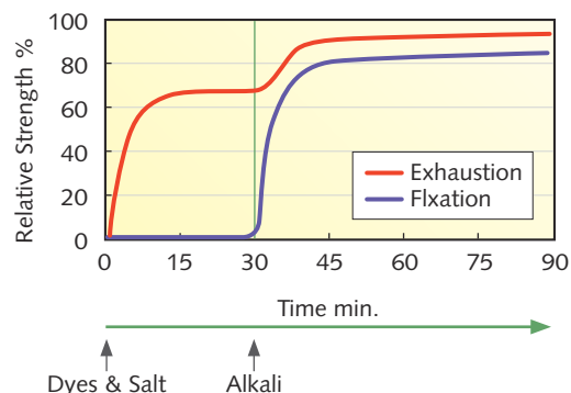
吸盡固著曲線 Exhaustion & Fixation
