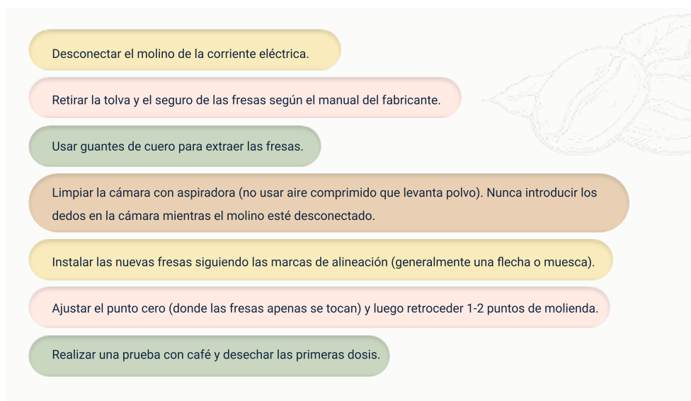
Figura 1. Procedimiento seguro para cambiar las fresas del molino
