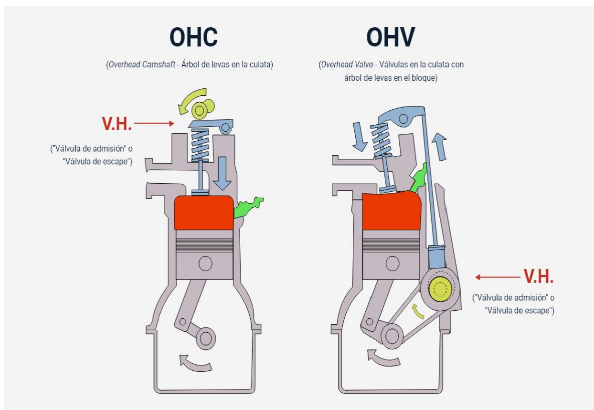
Figura 13. Esquema comparativo de configuraciones OHV y OHC
