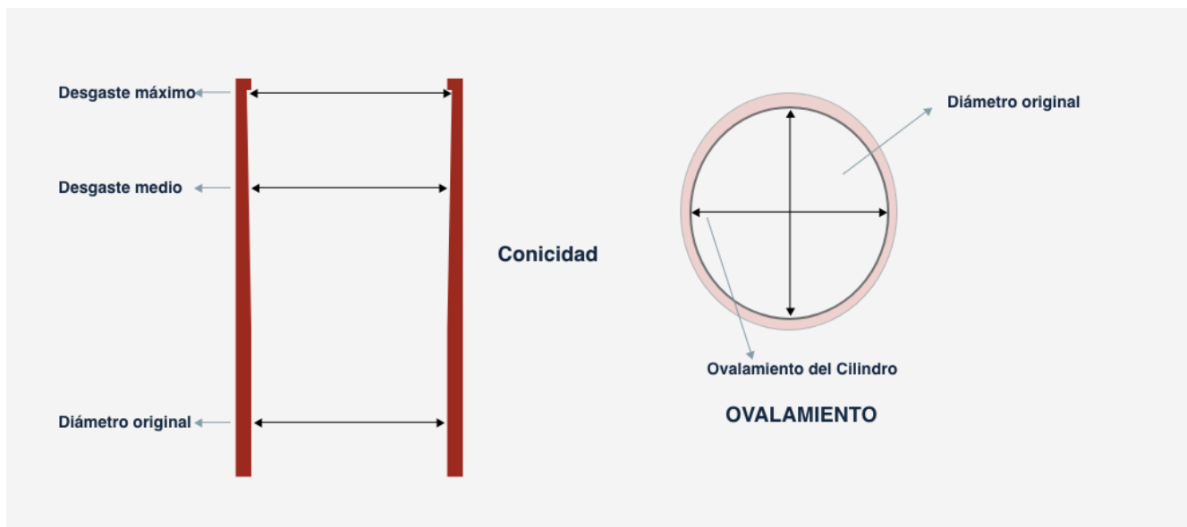
Figura 6. Análisis de desgaste y deformaciones en cilindros: parámetros críticos para rectificación
