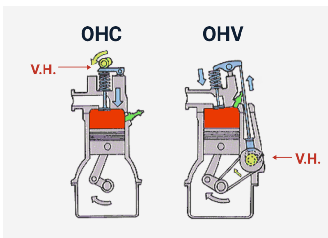
Figura 13. Esquema comparativo de configuraciones OHV y OHC.
