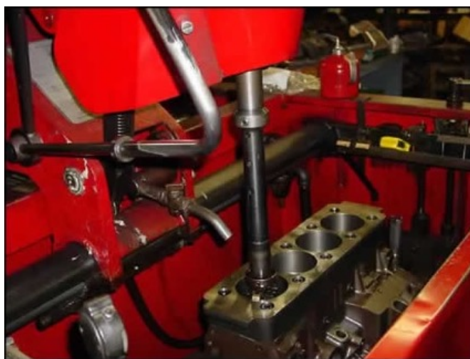
Figura 9. Proceso de acabado superficial por bruñido en cilindro.
