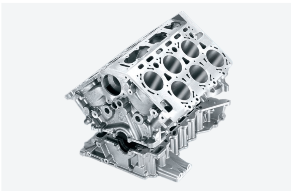
Figura 2. Bloque de cilindros y sus materiales.
