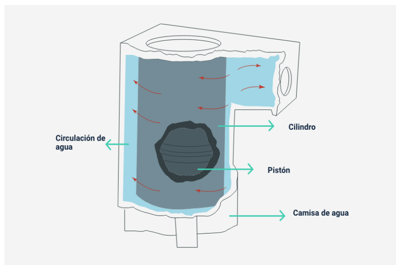
Figura 5. Corte de bloque con camisa húmeda y circulación de refrigerante.
