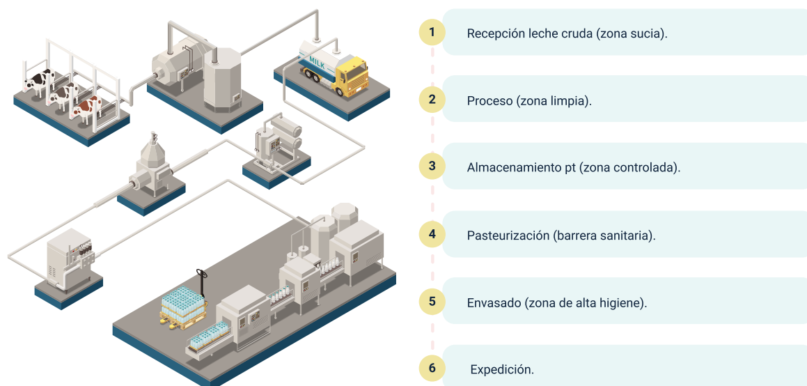
Figura 3. Flujo unidireccional en planta láctea
