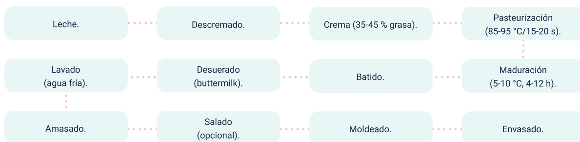
Figura 6. Diagrama de flujo de mantequilla
