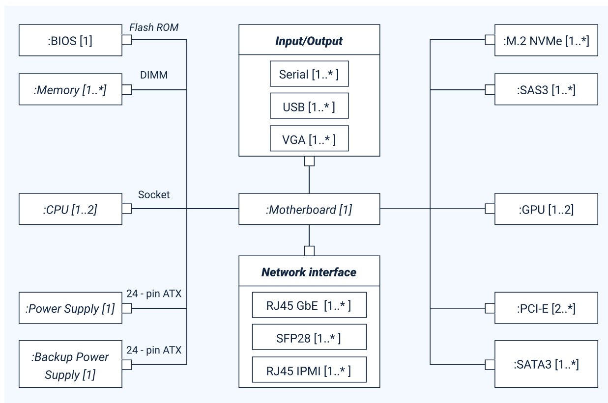
Figura 2. Diagrama de componentes de la arquitectura de hardware de un computador
