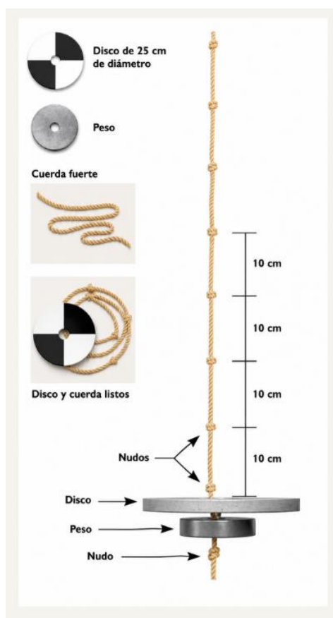
Figura 6. Construcción artesanal de un disco Secchi
