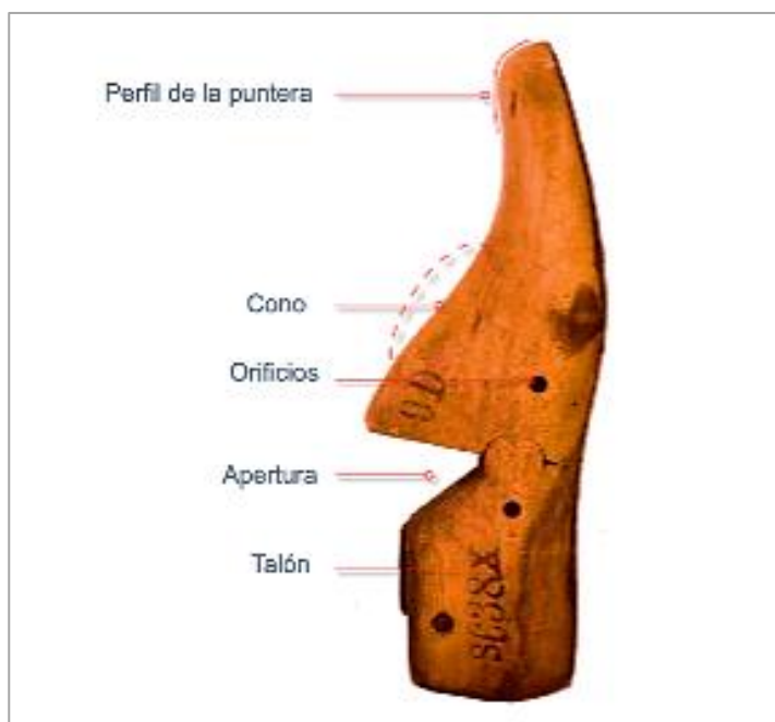
Figura 5. Perfil lateral de la horma con elementos constructivos
