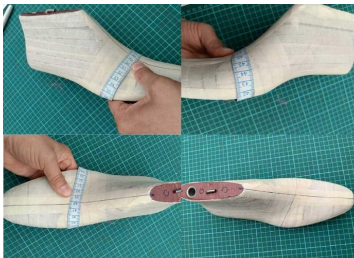
Figura 3. Trazado de la línea metatarsiana
