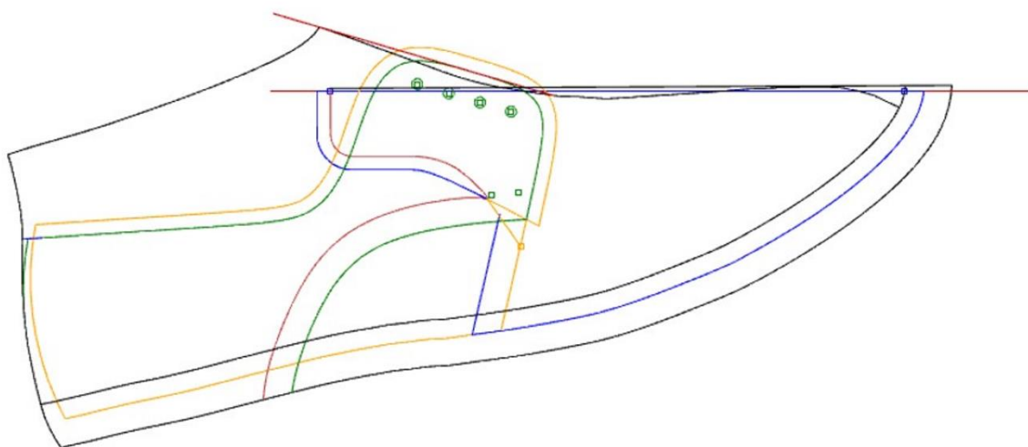
Figura 36. Reducción del forro-capellada sobre el eje
