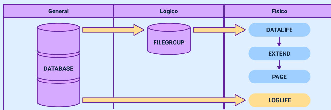
Figura 6. Arquitectura de un DBMS
