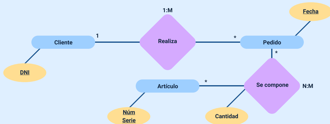
Figura 8. Ejemplo modelo entidad-relación
