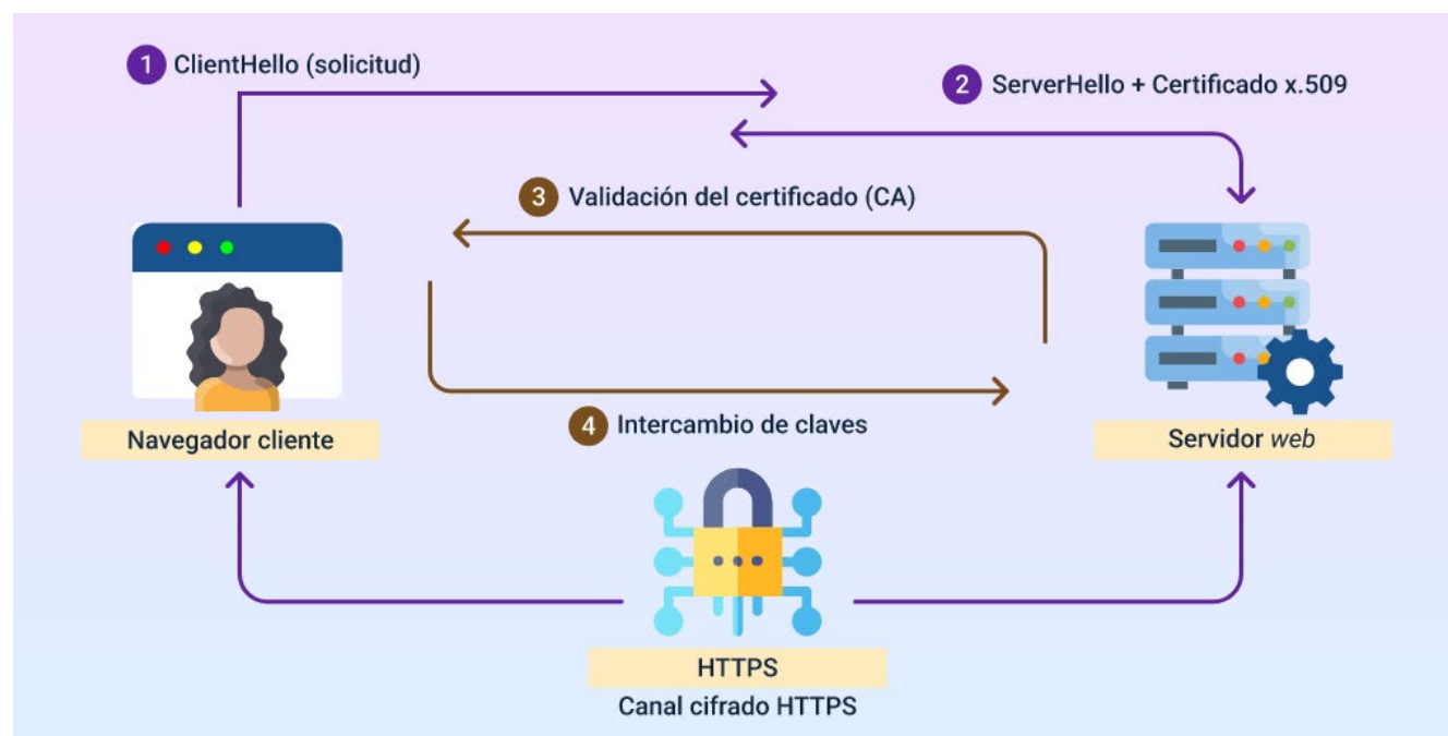
Figura 3. Diagrama de secuencia del apretón de manos HTTPS
