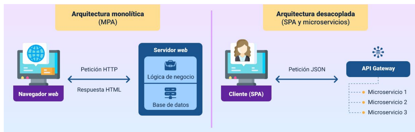
Figura 1. Esquema de arquitecturas web principales (monolítica vs. desacoplada con SPA)
