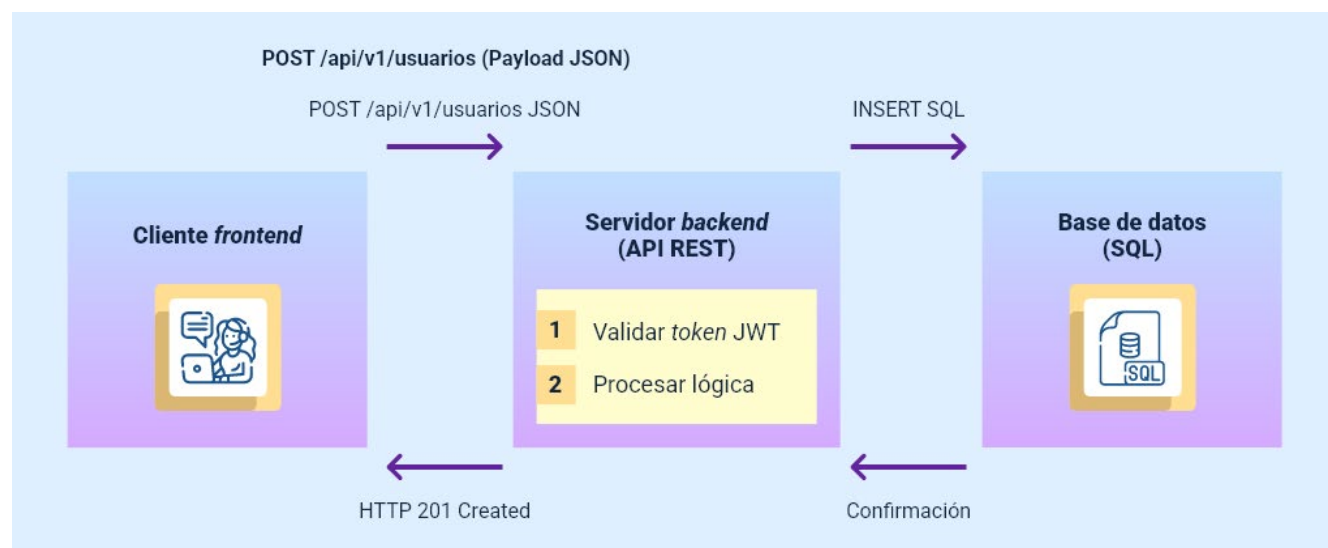
Figura 4. Diagrama de interacción cliente - API REST - base de datos
