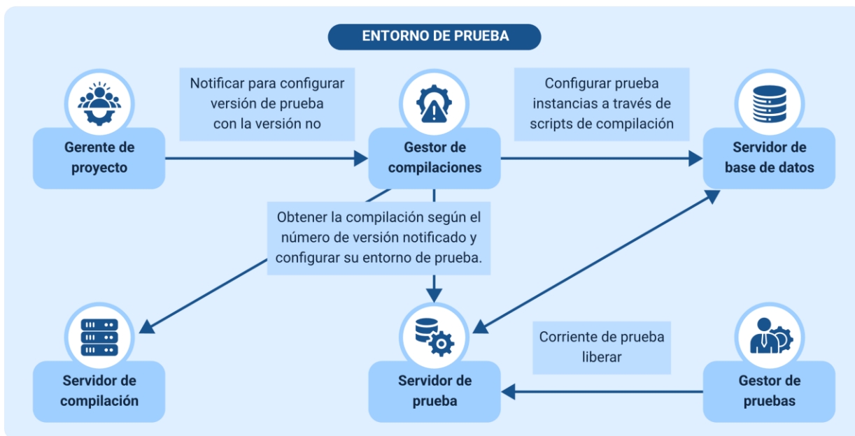
Figura 6. Asignación y distribución de recursos en el proceso de pruebas de software.
