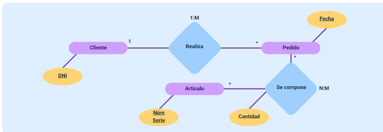
Figura 8. Ejemplo modelo entidad-relación
