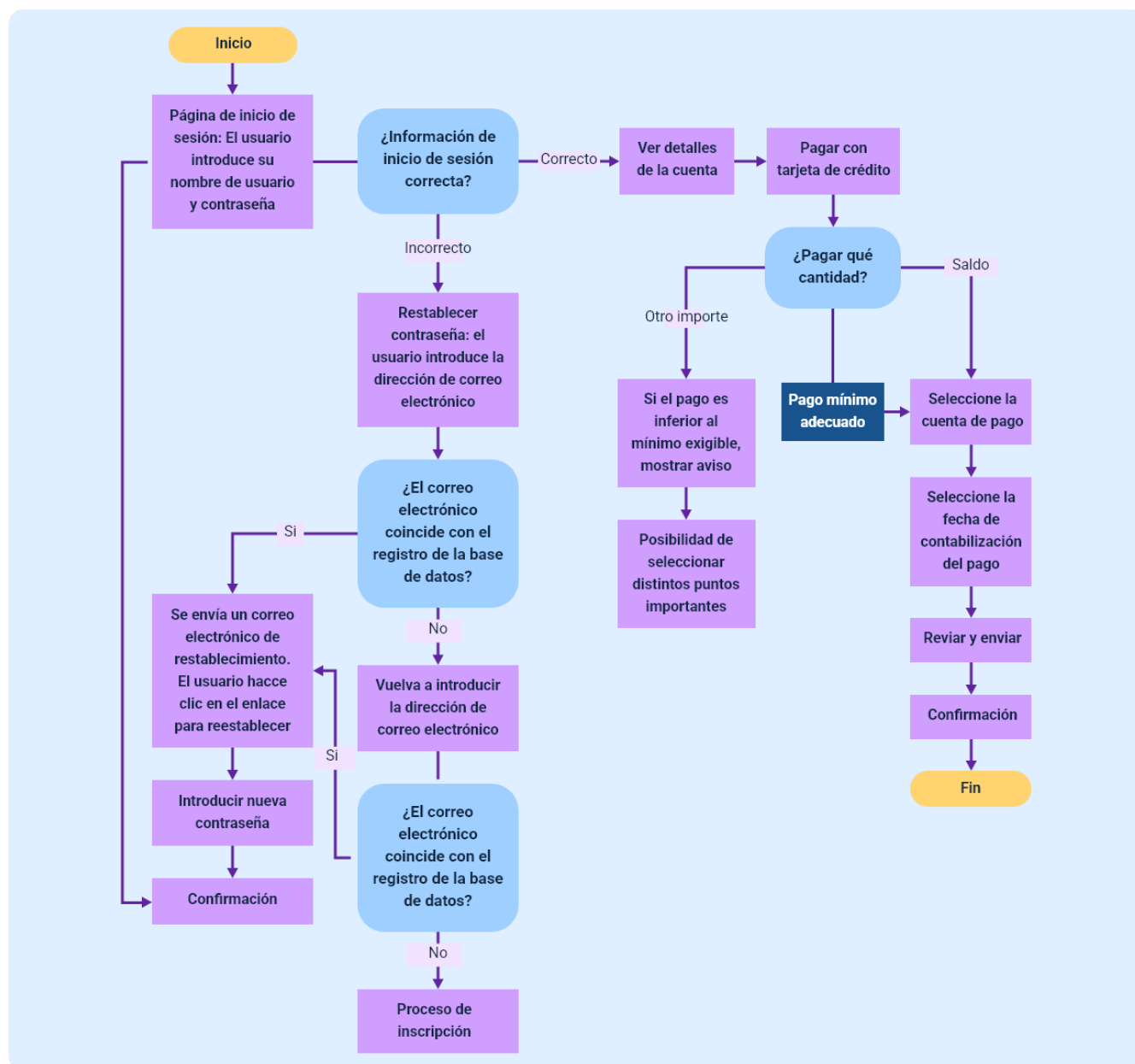
Figura 7. Interacción usuario – DBMS – base de datos
