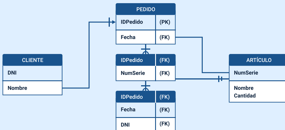
Figura 9. Ejemplo_modelo_lógico
