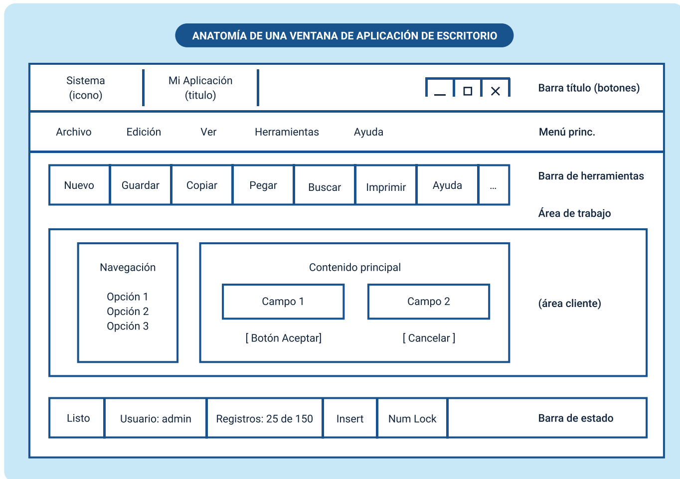
Figura 2. Anatomía de una aplicación de escritorio típica (Windows)
