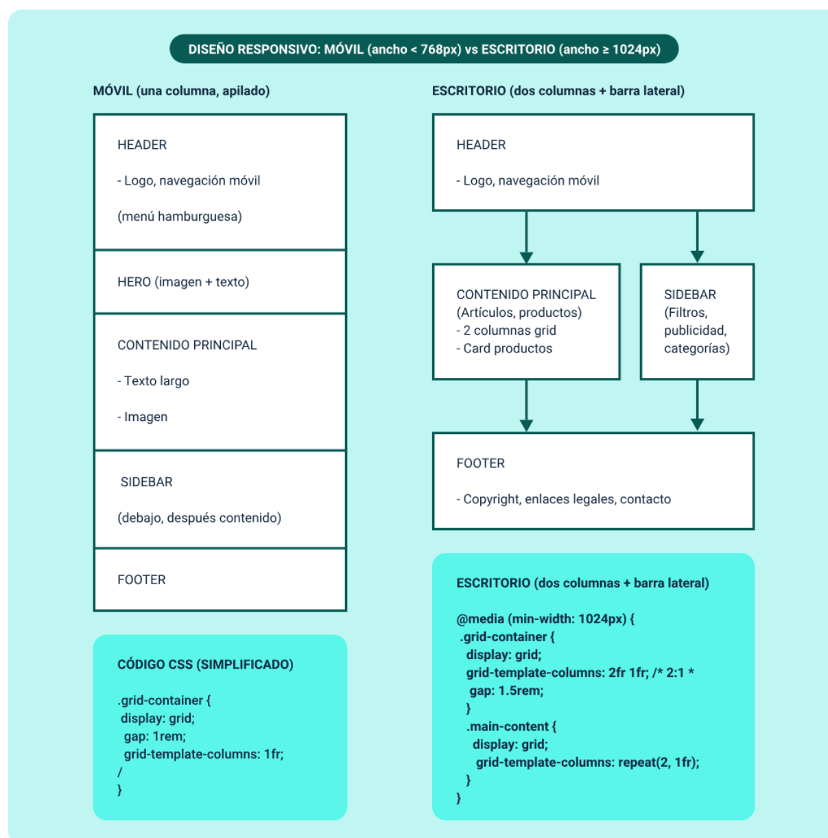
Figura 4. Diseño responsivo con CSS Grid y Flexbox en dispositivos móviles y de escritorio
