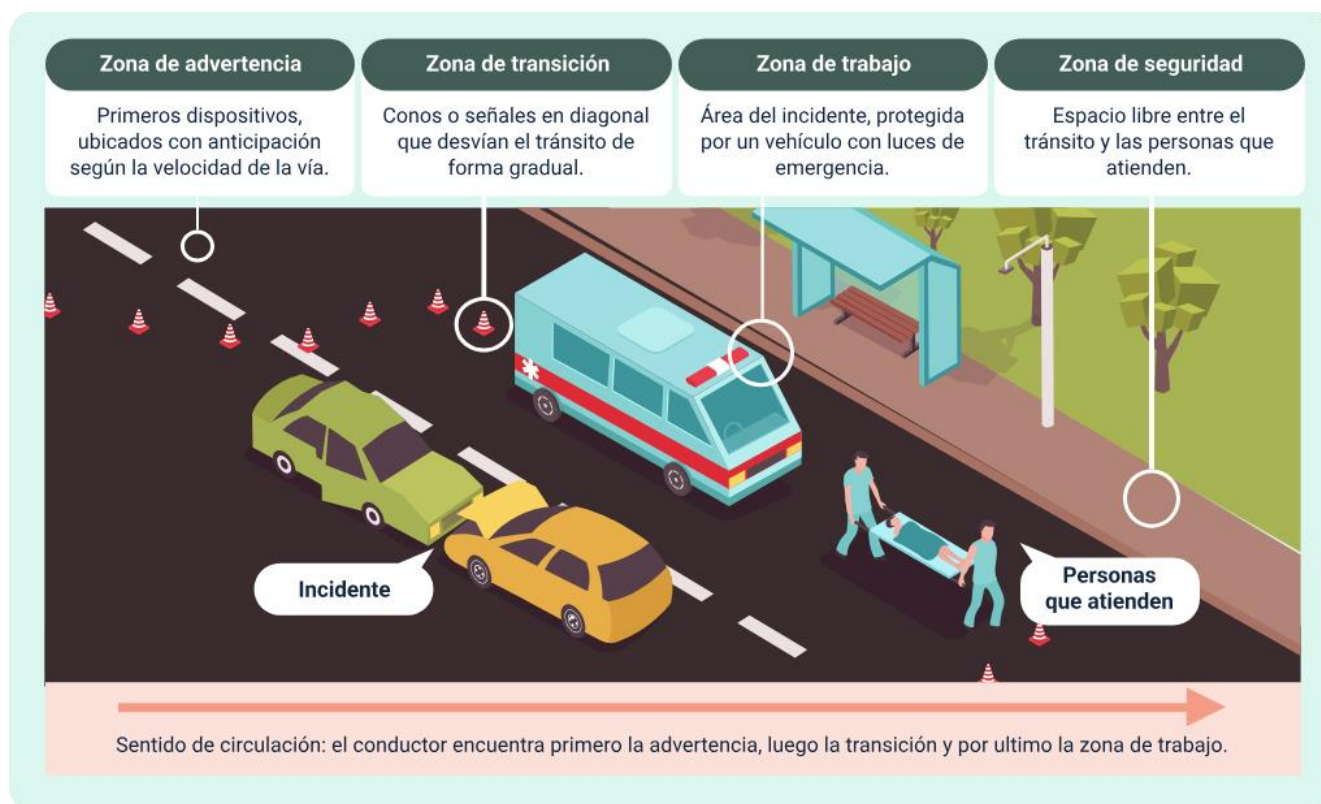
Figura 1. Disposición del balizaje en una vía
