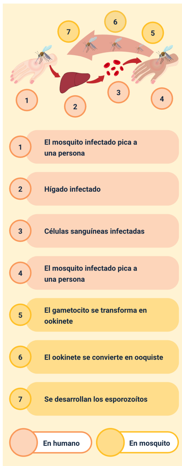
Figura 6. Proceso de la malaria
