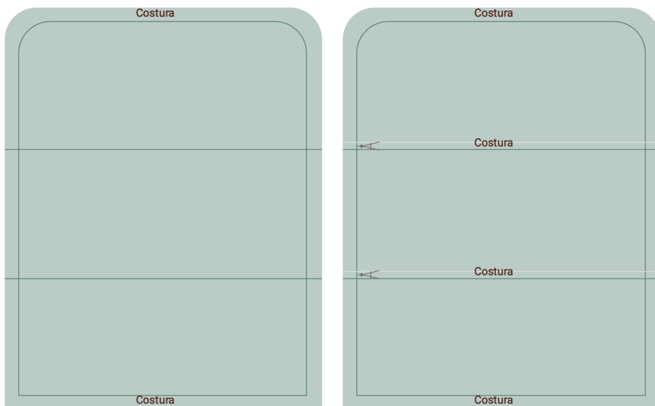
Figura 33. Molde porta documentos
